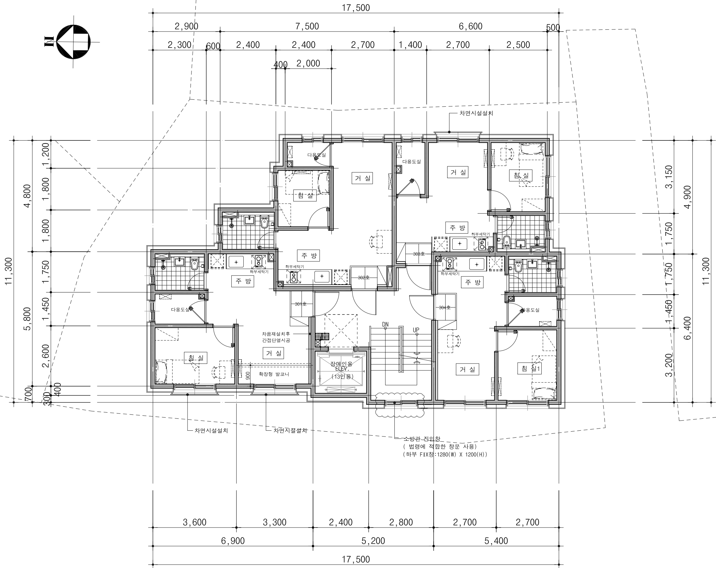
3 층 평 면 도 축척 : 1/100
